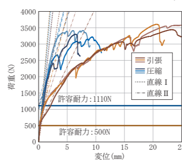
野縁方向一方向加力グラフ
