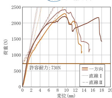
一方向加力グラフ
