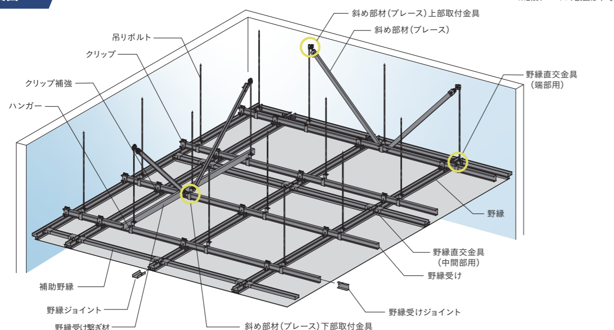
天井姿図
