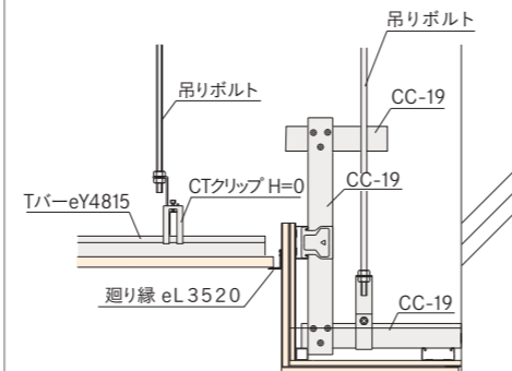
■下り天井の納まり ①
