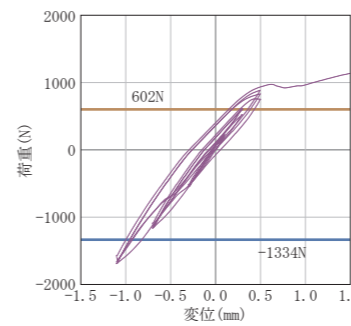
野縁方向繰り返し加力グラフ
