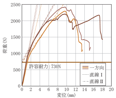
一方向加力グラフ
