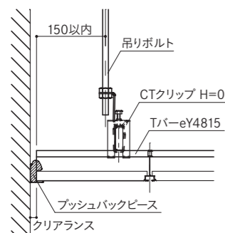
■壁際との納まり例 1-① (プッシュバックピースのみを使用した場合)
