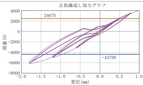
斜め部材 AS-25(25×19×5×1.0)
