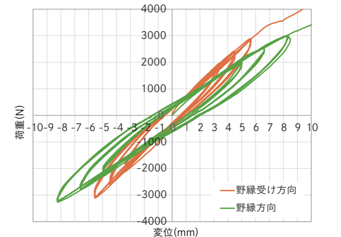
JIS19形仕様 60度 繰り返し加力
