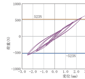
野縁受け方向繰り返し加力グラフ
