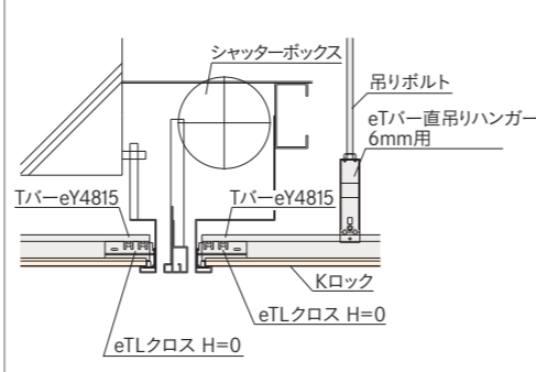
■シャッターボックスの納まり
