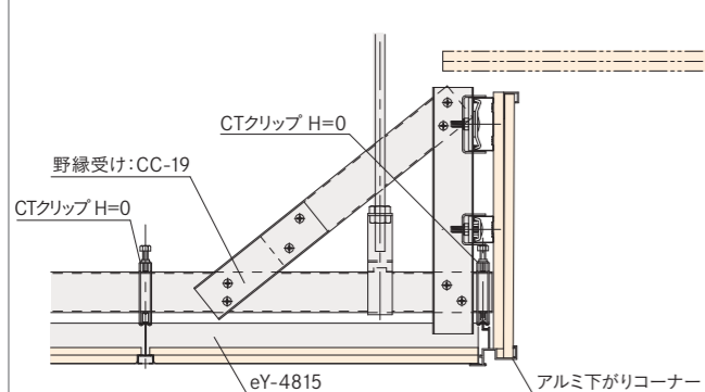
■下り天井の納まり ②
