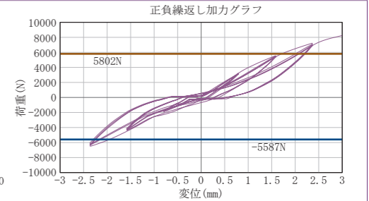
斜め部材 C-60×30×10×1.6
