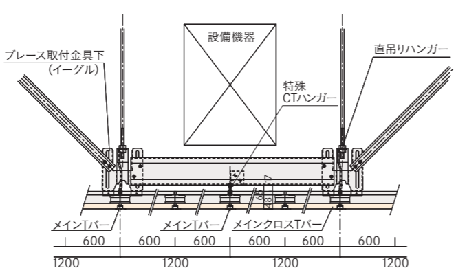
■設備機器周りの補強例
