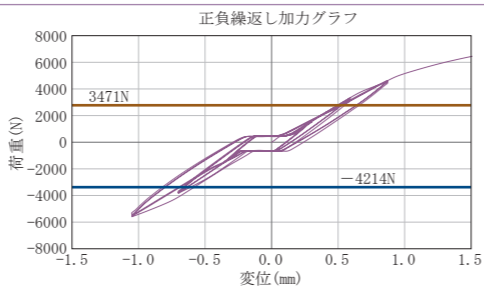
斜め部材 C-60×30×10×1.6
