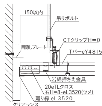
■壁際との納まり例 3
