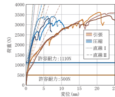
野縁方向一方向加力グラフ
