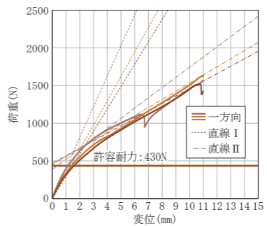
野縁受け方向一方向加力グラフ
