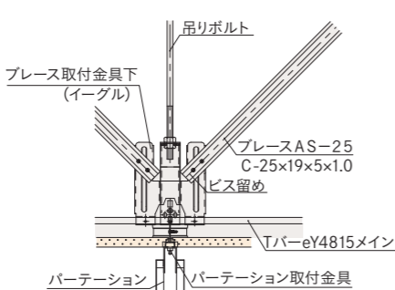
■eY4815 パーテーション設置部
