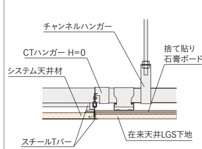
■在来天井との納まり
