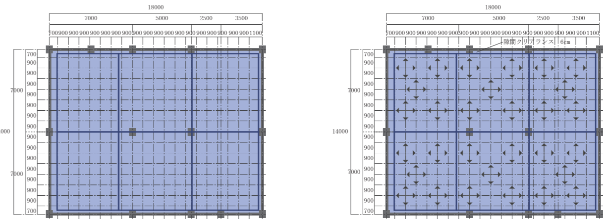
斜め部材選定の目安表 (JIS19 形仕様)
