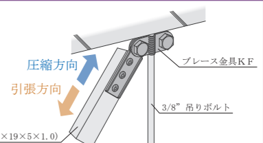
斜め部材 AS-25(25×19×5×1.0)
