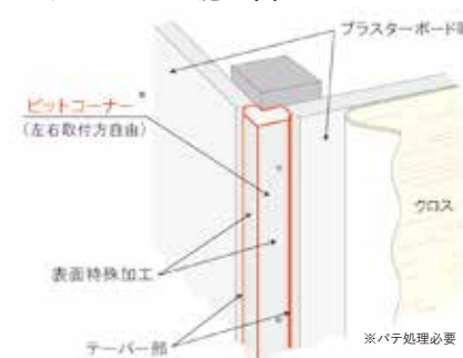
ピットコーナー施工図
