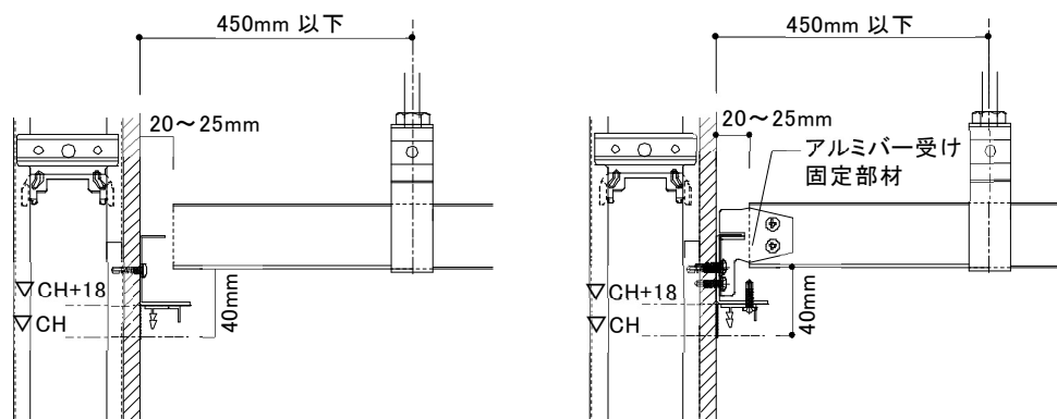
図 2-6-2 アルミバー受け固定部材の施工手順(壁面が軽量鉄骨の場合)
