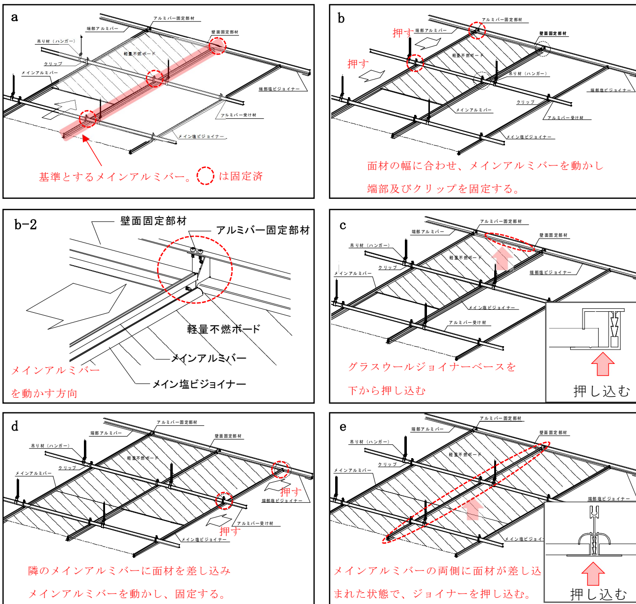
図 2-8-3 施工手順
