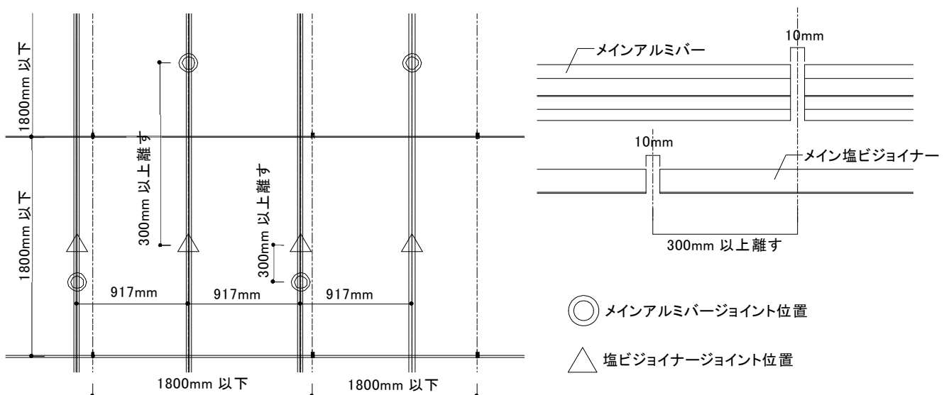
図 2-7-8 メイン塩ビジョイナージョイントの千鳥配置
