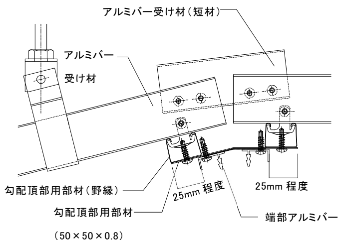
図 2-10-9 勾配頂部端部アルミバー取付け
